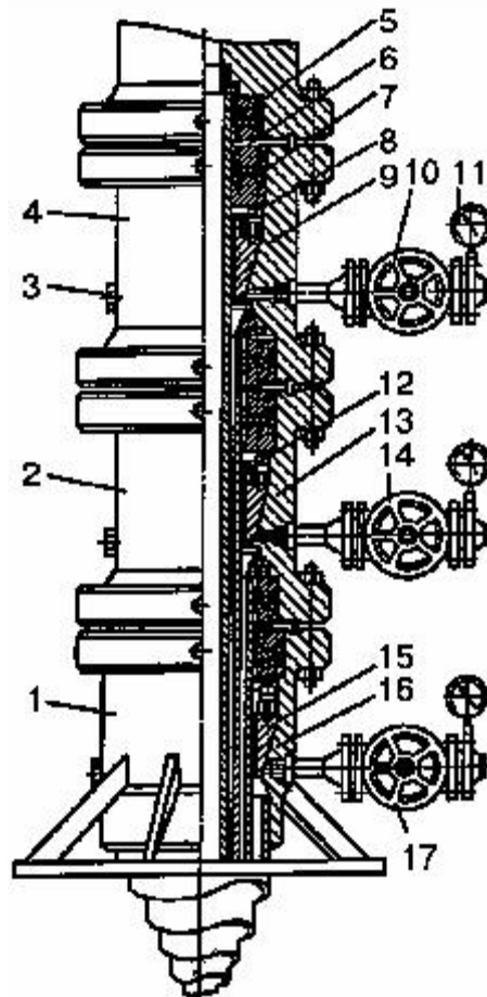
Рисунок 2.1 - трикорпусні колонна обв'язка ОК
