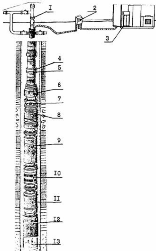
Рисунок 9.1 - Встановлення занурювального відцентрового насоса:
