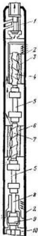
Рисунок 10.2 - Схема гвинтового свердловинного насоса
