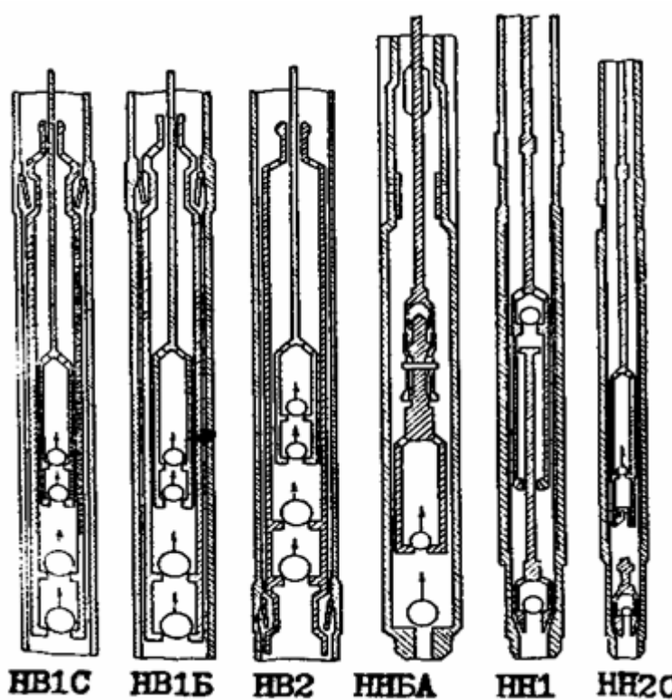
Рисунок 5.3 - Типи свердловинних штангових насосів
