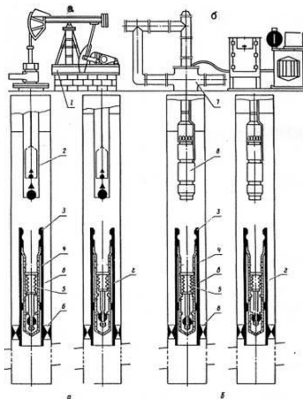
Рисунок 10.5 - Комплекс обладнання типу КОС:
