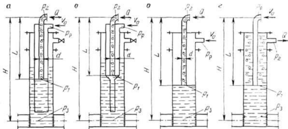
Рисунок 4.1 - Конструкції і системи газліфтних підйомників: a Б В - відповідно дво-, півтора- і однорядні підйомники кільцевої системи; г - однорядний підйомник центральної системи
