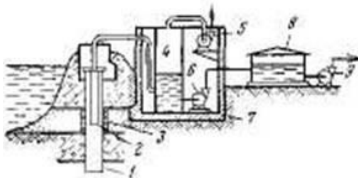
Рисунок 13.1 - Схема водозаборів:
