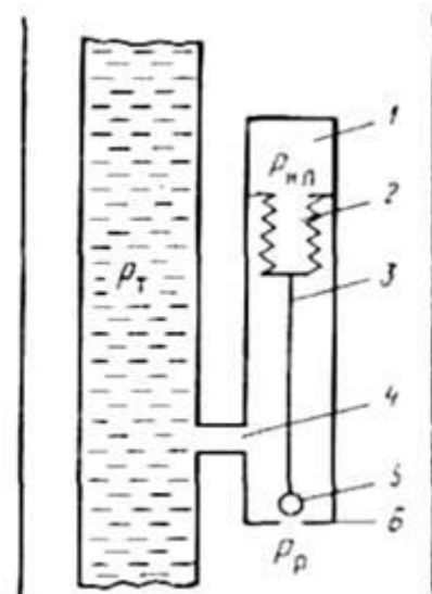
Рисунок 4.3 - Газліфтний клапан, який працює від тиску газорідинний середовища
