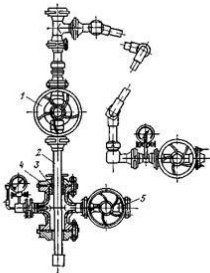
Рисунок 15.1 - Гирлова арматура АП-65-150
