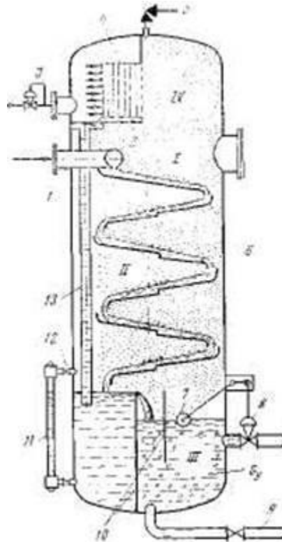
Рисунок 17.1 - Пристрій вертикального сепаратора:
