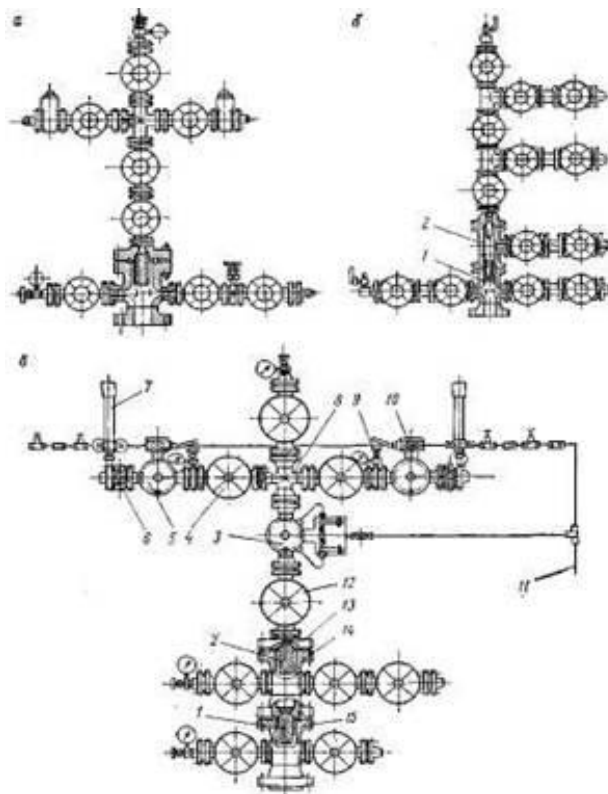
Рисунок 3.3 - Фонтанна арматура:
