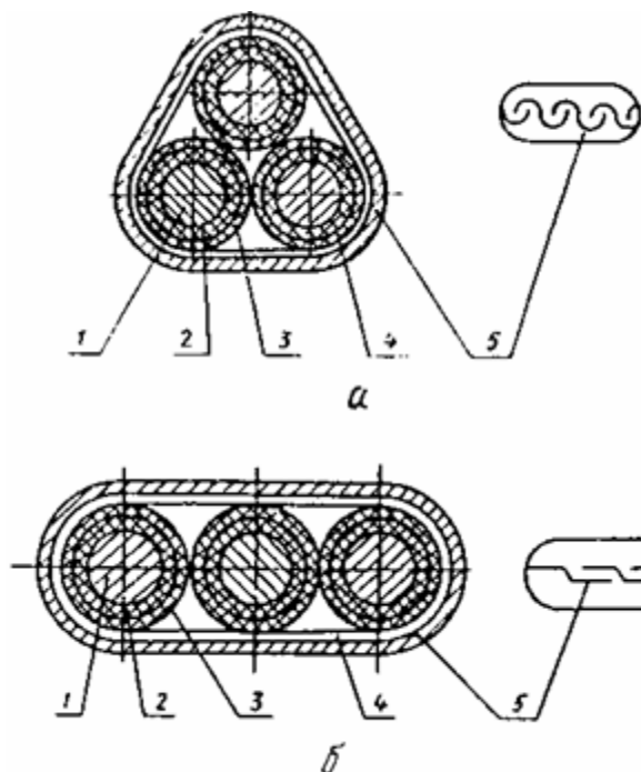
Рисунок 9.6 - Кабелі:
