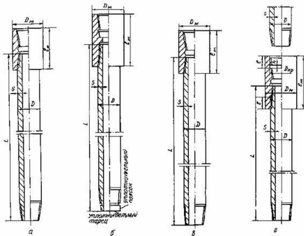
Рисунок 2.2 - Труби насосно-компресорні муфтові гладкі а- з конічною різьбою трикутного профілю; б - з конічною різьбою трапецеїдального профілю; в - з конічною різьбою трикутного профілю з підвищеною пластичністю і морозостійкості; г - з конічною різьбою трикутного профілю з вузлом ущільнення з полімерного матеріалу
