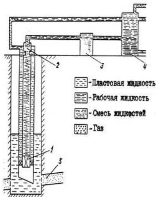
Рисунок 8.2 - Струйно-насосна установка
