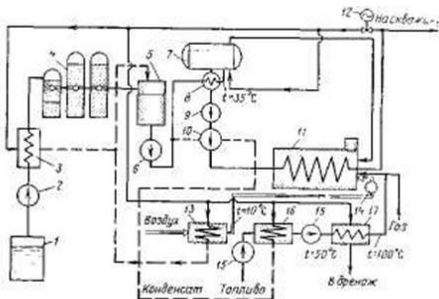
Рисунок 15.3 - Схема парогенераторної установки ППГУ-4 / 120М
