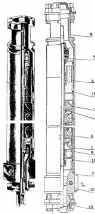
Рисунок 9.2 - Модуль секція насоса:
