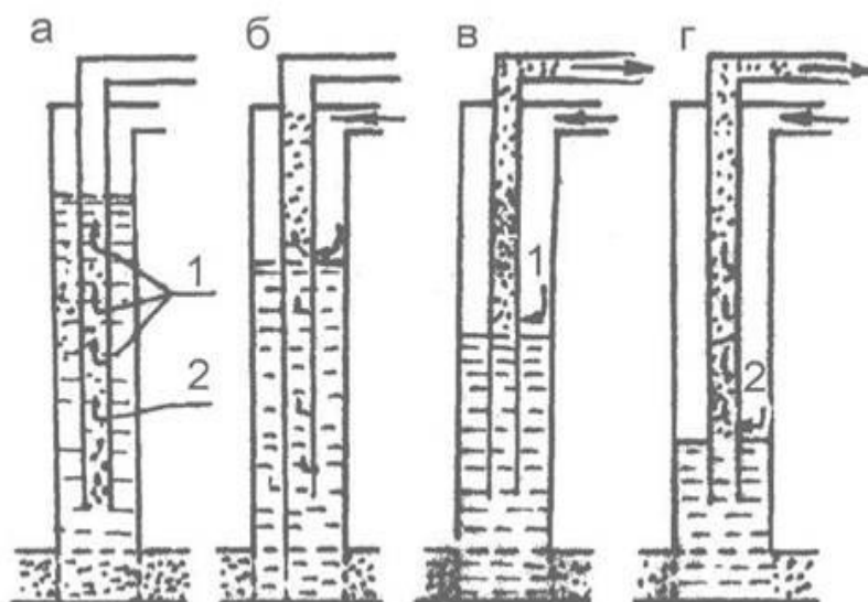
Рисунок 4.2 - Процес запуску газліфтної свердловини 1 - муфти з отворами для пуску свердловини; 2 - муфта з отворами для роботи свердловини
