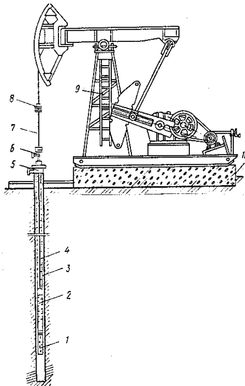
Рисунок 5.1 - Схема установки штангового свердловинного насоса
