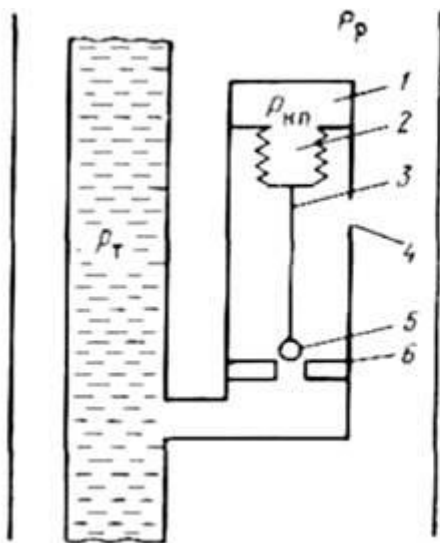
Рисунок 4.2 - Газліфтний клапан, який працює від робочого тиску
