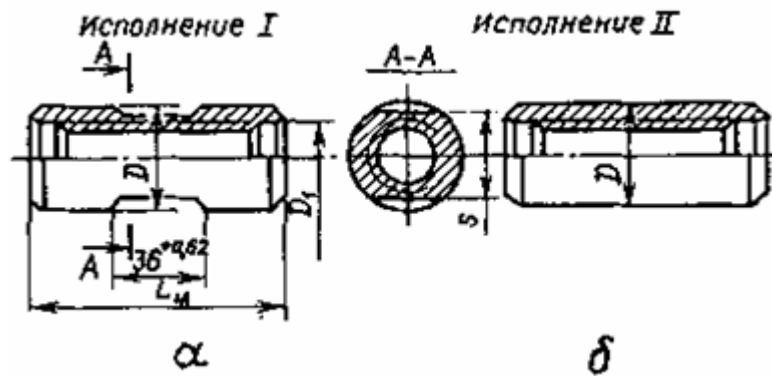
Рисунок 5.6 - Сполучна муфта: а - виконання I; б - виконання II
