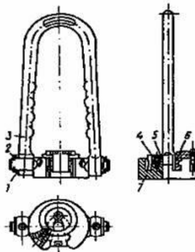
Рисунок 12.4 - Елеватор штанговий ЕШН
