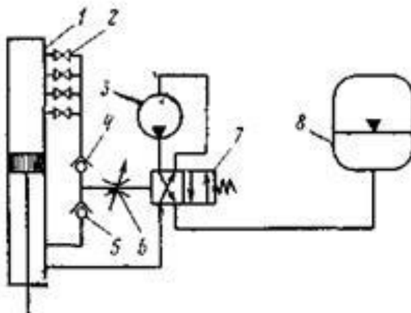
Рисунок 7.1 - Установка з закритою гідравлічною схемою
