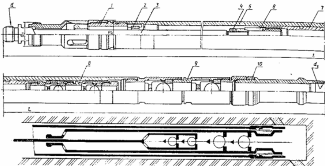
Рисунок 5.4 - свердловини штанговий насос виконання НВ2Б:
