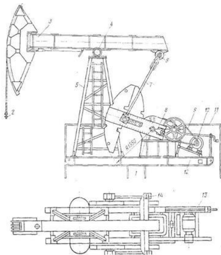
Рисунок 6.2 - Загальний вигляд верстата-качалки
