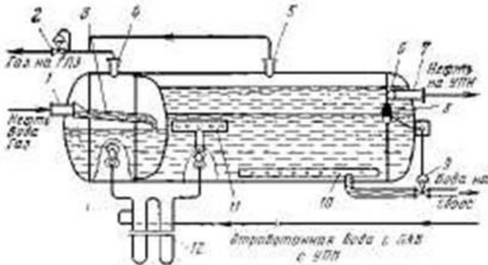
Рисунок 17.2 - Горизонтальний трифазний сепаратор:
