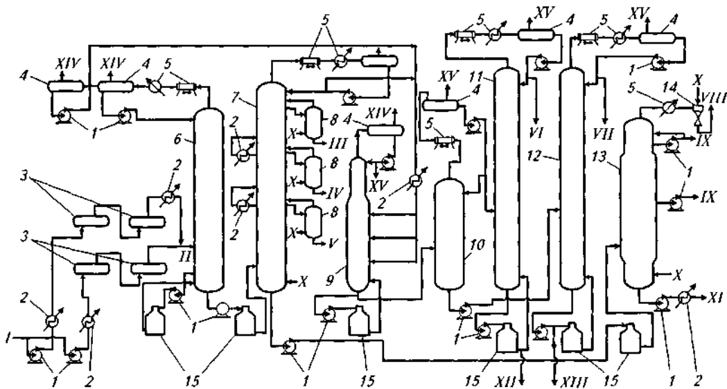
Рисунок 7.2 - Установка з комбінованою схемою
