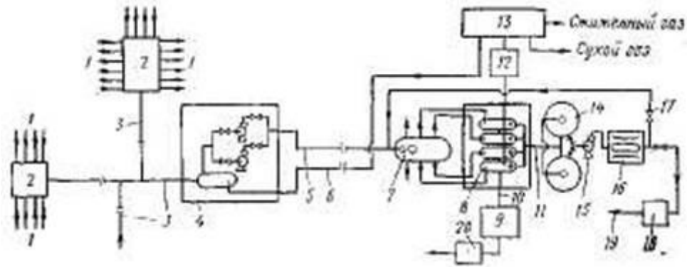
Рисунок 16.3 - Високонапірна система збору продукції свердловин на великих родовищах:
