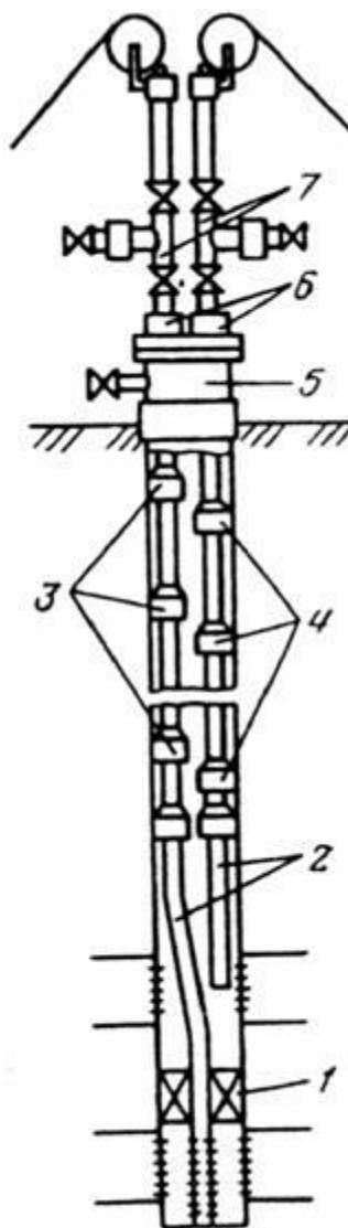
Рисунок 11.1 - Схема установки для роздільної експлуатації двох пластів з двома паралельними рядами труб за схемою фонтан-фонтан:
