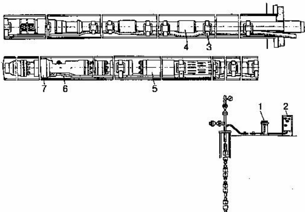
Рисунок 10.1 - Установки занурювального гвинтового здвоєного електронасоса
