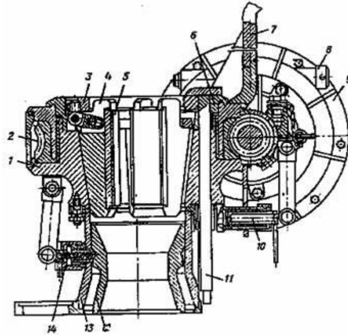
Рисунок 12.5 - Автомат АПР-2ВБМ
