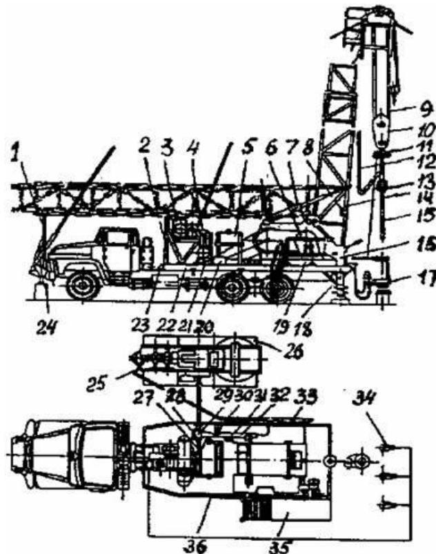
Рисунок 12.3 - Агрегат А-50М
