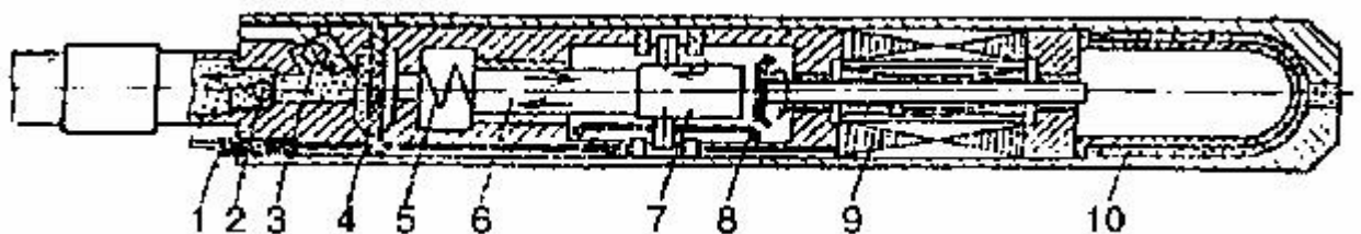
Рисунок 10.3 –Занурювальний діафрагмовий електронасос:
