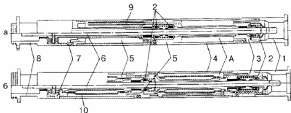
Рисунок 9.5 - Гідрозахист:
