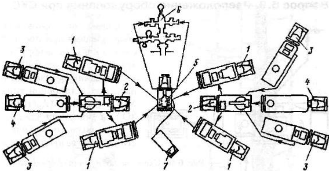
Рисунок 14.3 - Схема розташування обладнання при проведенні гідророзриву пласта: 1 - насосний агрегат 4АН-700; 2 - піскозмішувальний агрегат; 3 - автоцистерна; 4 - пісковоз; 5 - блок манифольда 1БМ-700; 6 - арматура гирла 2АУ-700; 7 - станція контролю і управління процесом
