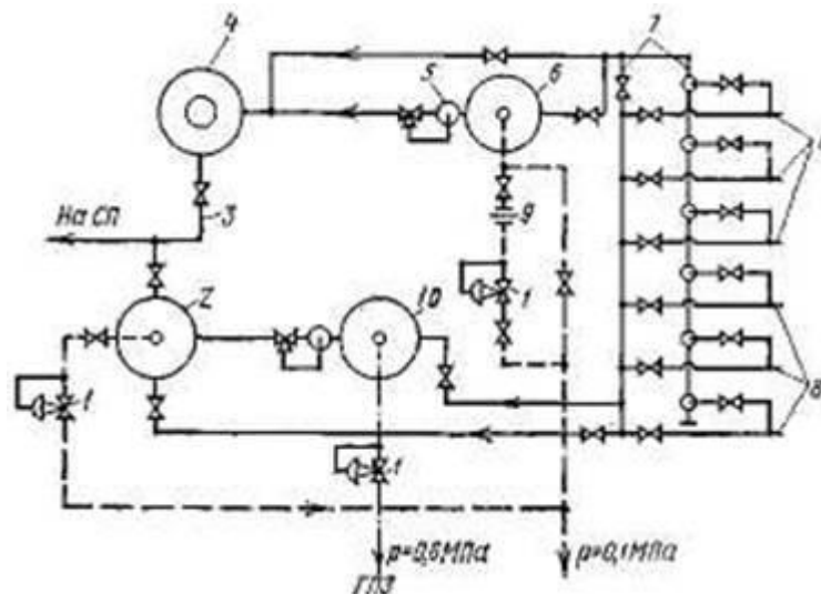
Рисунок 16.2 - Групових замір-сепарації установка:
