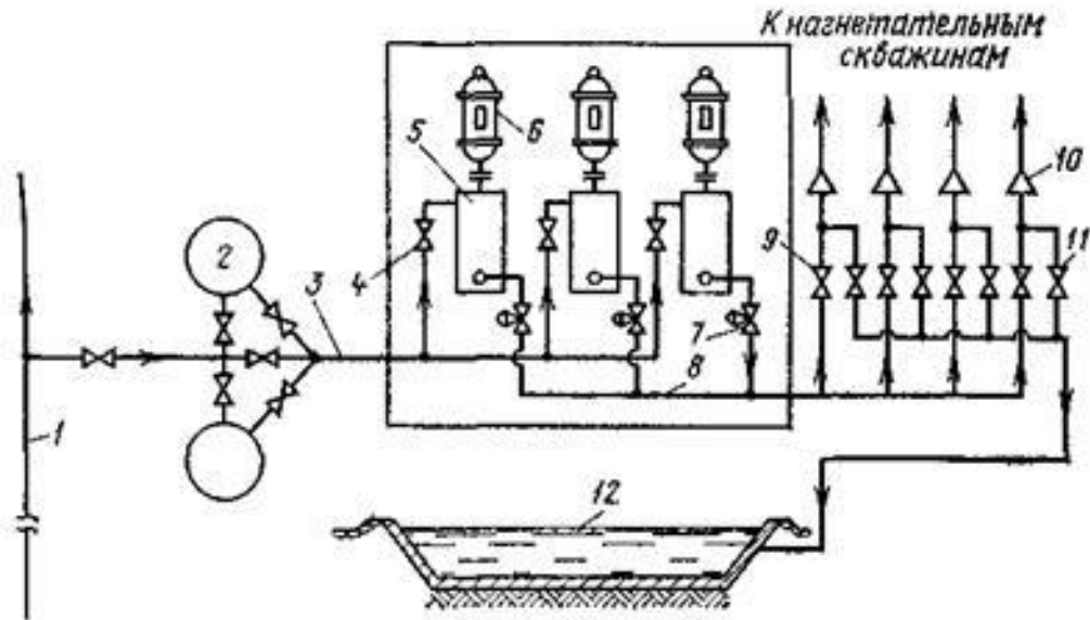
Рисунок 13.3 - Схема блокової КНС:
