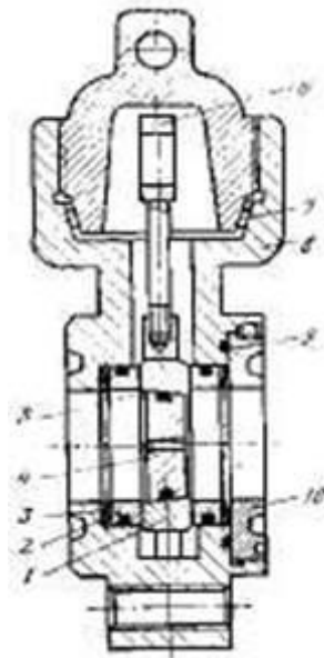
Рисунок 3.5 - Швидкозмінний штуцер:
