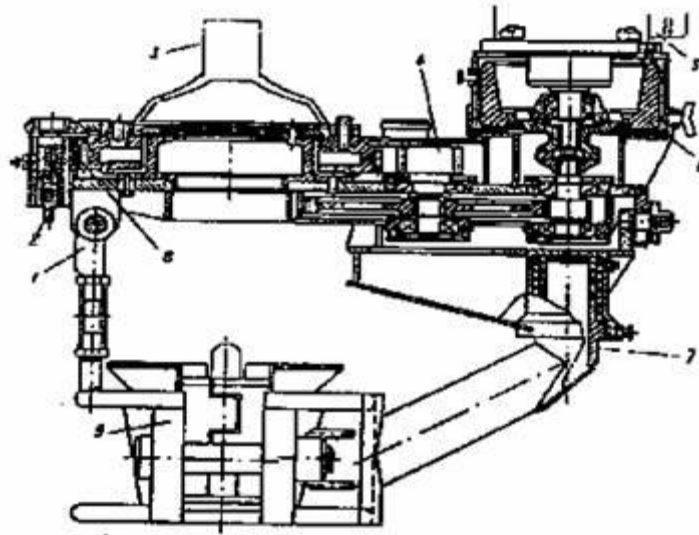
Рисунок 12.6 - Ключ механічний універсальний КМУ-50
