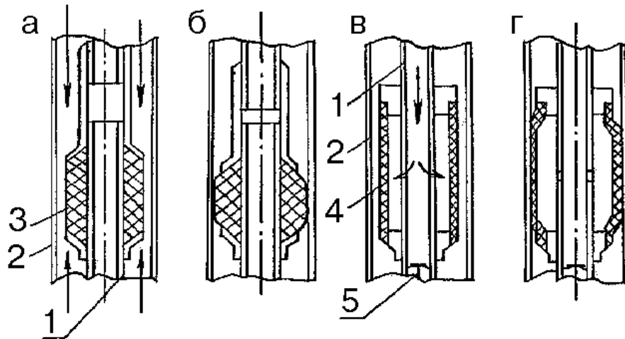
Рис. 3. Пакера
