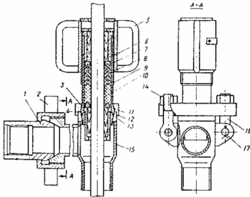
Рисунок 6.1 - гирлового сальника типу СУС1
