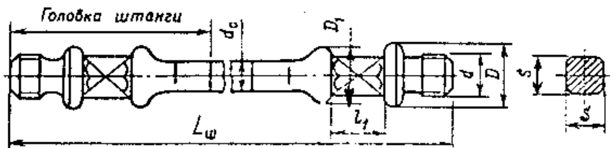
Рисунок 5.5 - Насосна штанга
