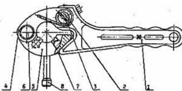
Рисунок 12.8 - Ключ трубний КТЛ
