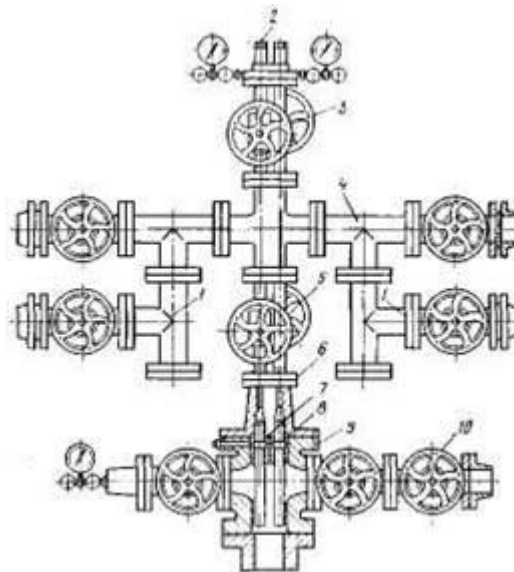
Рисунок 11.2 - Загальний вигляд двоєної фонтанної арматури
