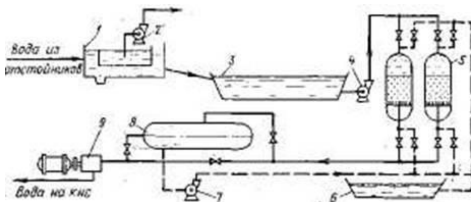
Рисунок 13.2 - Відкрита схема установки очищення стічних вод: 1- нафтоуловлювач; 2 - нафтовий насос; 3 - відстійник; 4 - насос; 5 - піщані фільтри; 6- відстійник для забрудненої води; 7 - насос для проведення промивки фільтрів; 8- ємність для чистої води; 9 - насос для подачі води на КНС
