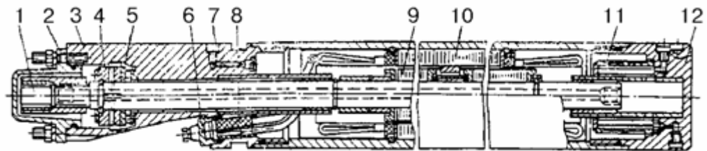
Рисунок 9.4 - Електродвигун серії педу:
