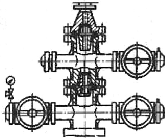
Рисунок 3.2 - Трубна головка:
