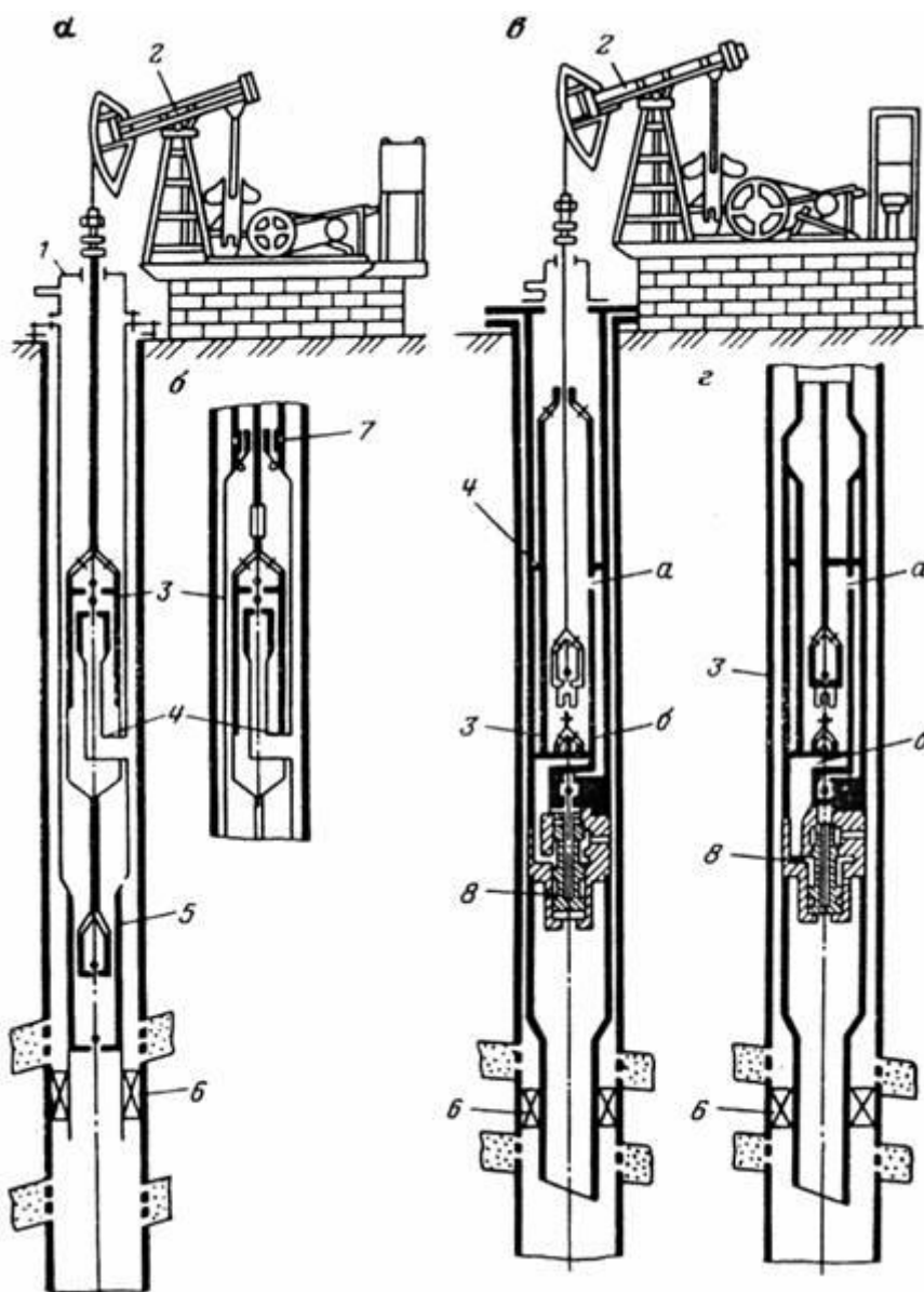
Рисунок 11.2 - Установки для ОРЕ двох пластів свердловинами, обладнаними штанговими свердловинними насосами:
