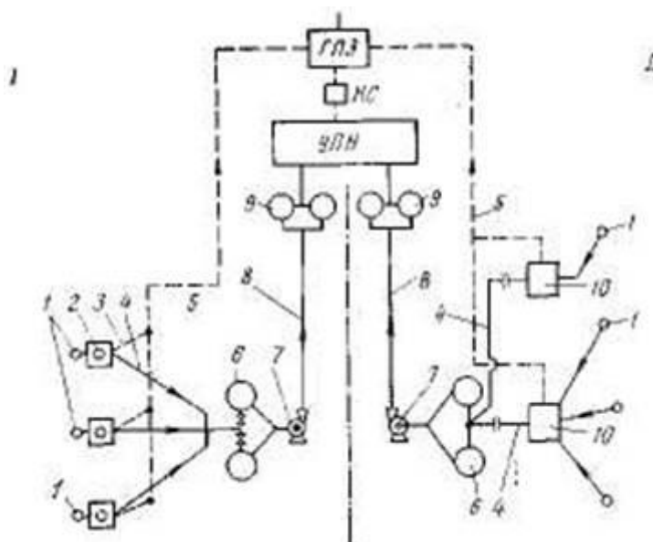
Рисунок 16.1 - Схема самопливної двотрубної системи збору продукції свердловин:
