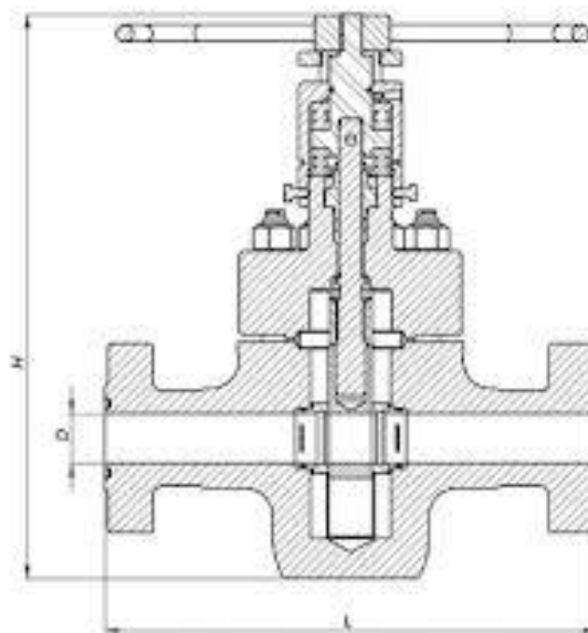
Рисунок 3.4 - Прямоточна плоскошіберна засувка
