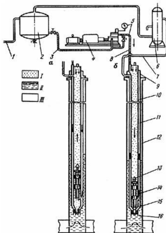
Рисунок 8.1 - Схема компонування обладнання гідропоршневим насосної установки
