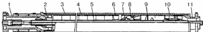
Рисунок 9.3 - Газосепаратор:
