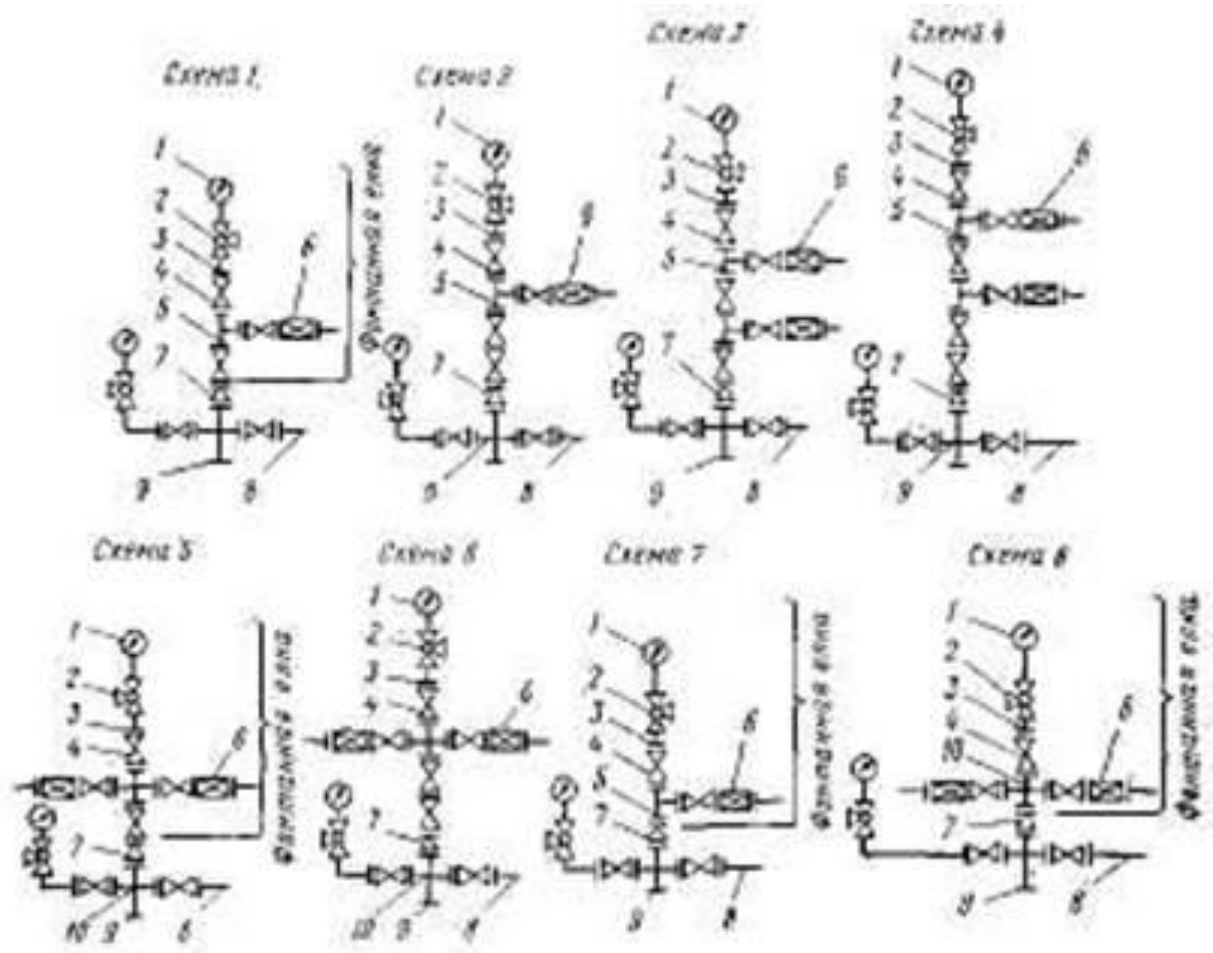
Рисунок 3.1 - Стандартизовані схеми фонтанних арматур:
