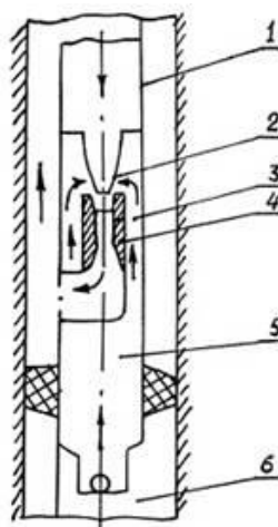
Рисунок 8.3 - Схема струминного насоса
