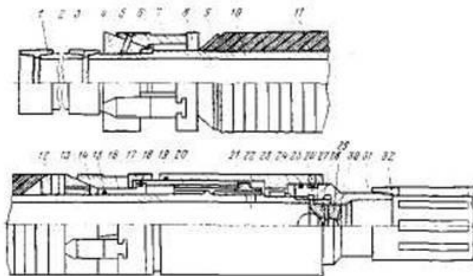
Рисунок 15.2 - Термостійкий пакер ПТГМ
