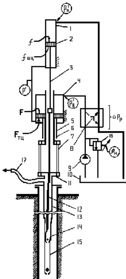
Рисунок 7.3 - Схема установки з використанням НКТ в якості врівноваження вантажу
