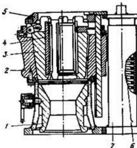
Рисунок 12.7 - Спайдер АСГ-80
